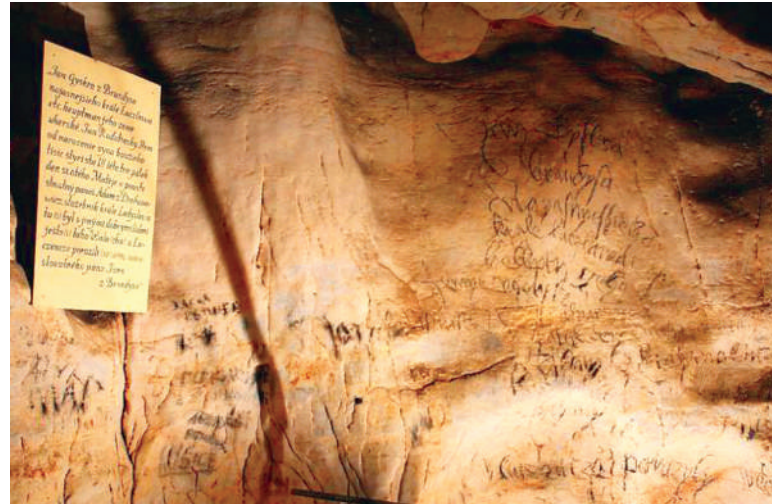
Foto: Kresby v jaskyni Domica
